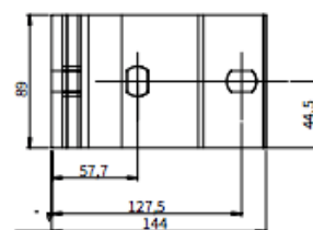
Bovenaanzicht plafondsteun
