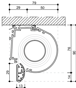
Plafondmontage
