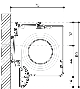
32.225.xx.xx Cassette Vierkant Wandmontage
